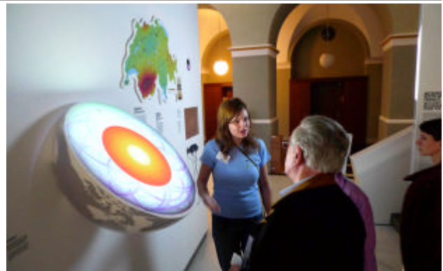
Aufprojektion zur Veranschaulichung der Mantelkonvektion im Erdinneren
